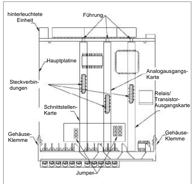
Ausgangskarten
