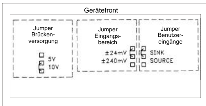
Jumper-Funktionen
